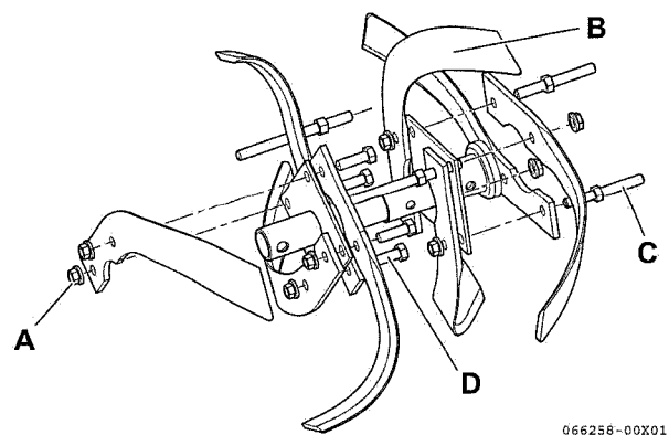
Eje de la cuchilla central e interior
