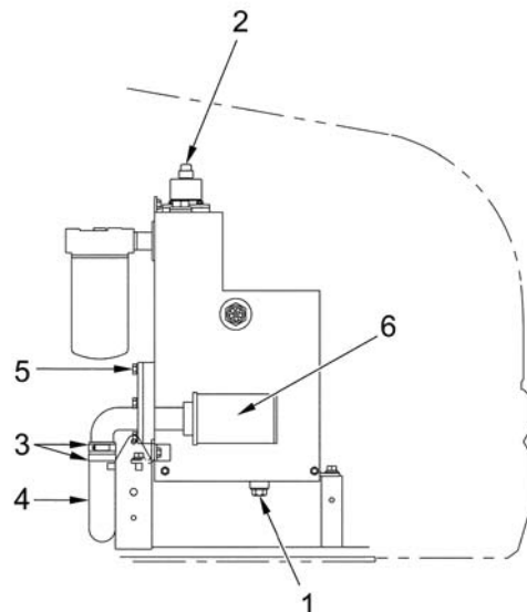
Posición de descarga del aceite hidráulico
