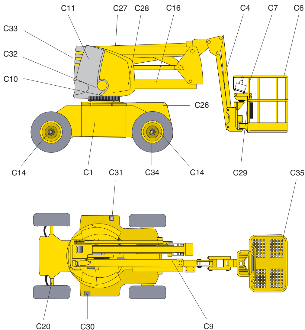
HA120PX - Designación de los componentes
