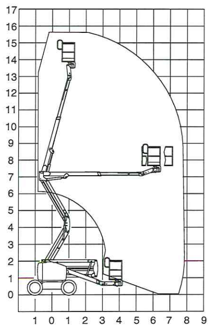
Cuadro de amplitud de movimientos de Z-45/25
