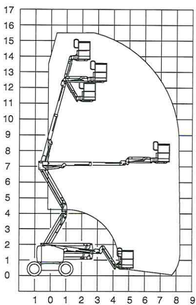
Cuadro de amplitud de movimientos de Z-45/25J
