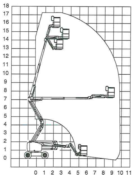
Cuadro de amplitud de movimientos de Z-51/30
