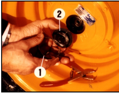
Fotografía 8 Desenganche
