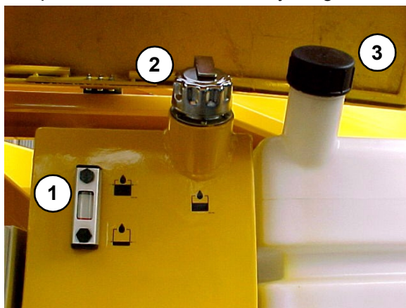
Fotografía 6 Depósito de aceite de motor y de gasóleo.
