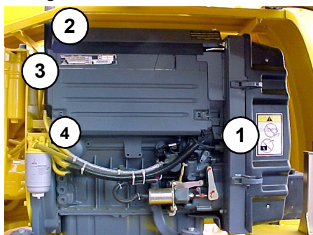
Fotografía 5 Motor
